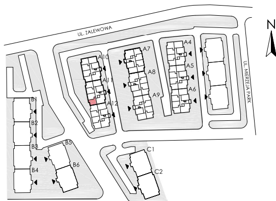
Schemat Zagospodarowania Terenu Szutowo, ul. Zalewowa
